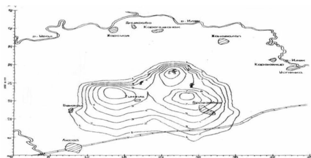
Рисунок 1 – Изолинии концентрации сернистого газа на уровне Z=2 м в момент времени t=16 ч 00 мин
