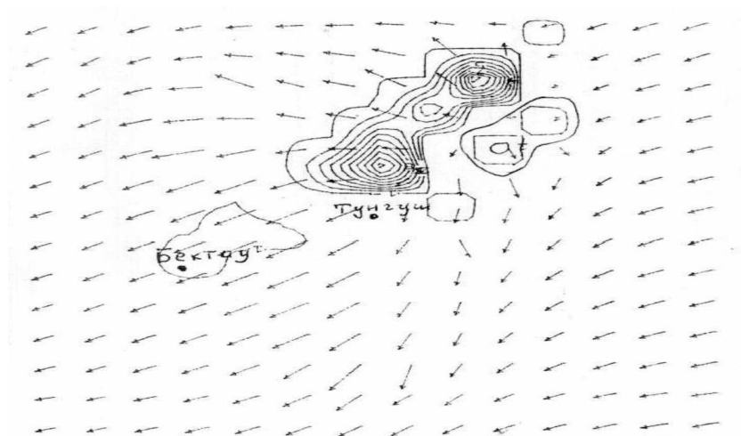
Рисунок 6а – Изолинии концентрации \text{NO}_2\text{b} поле вектора скорости на уровне Z=50 м в момент времени t=14 час. 00 мин
