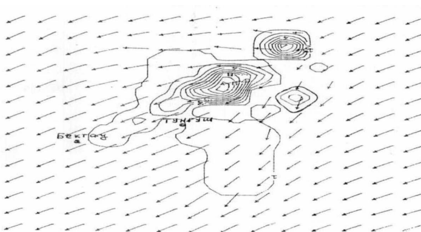
Рисунок 6б – Изолинии концентрации \text{NO}_2\text{b} поле вектора скорости на уровне Z=2 м в момент времени t=14 час. 00 мин.
