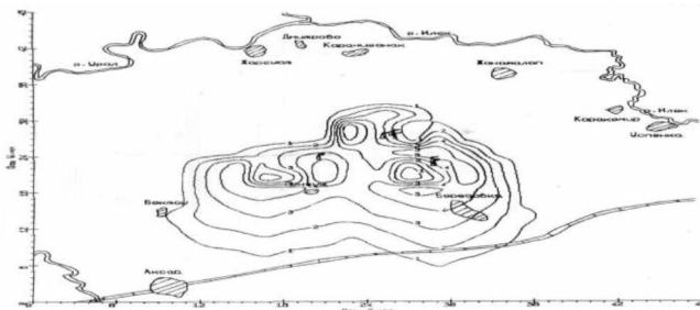
Рисунок 2 – Изолинии концентрации сернистого газа на уровне Z=2 м в момент времени t=7 час. 00 мин
