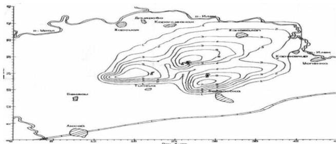
Рисунок 3 – Изолинии концентрации сернистого газа на уровне Z=2 м в момент времени t=16 час. 00 мин
