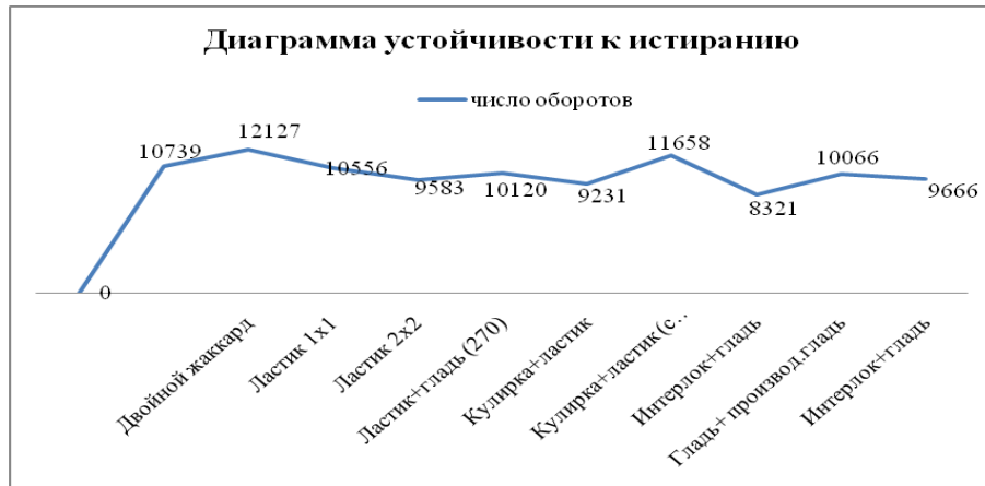
Рисунок 2 - Диаграмма показателей устойчивости к истиранию комбинированных переплетений.
