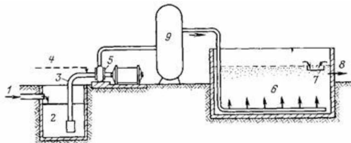
Сурет 3 - Ағынды флотацияға арналған құрылғының сызбасы 1-судың кіруі; 2-қабылдау резервуары; 3-соратын құбыр; 4-ауа құбыры; 5-су сорғыш; 6-флотациялық камера; 7-көбік жинағы; 8-тазаланған судың әкетілуі; 9-ағынды ыдыс
