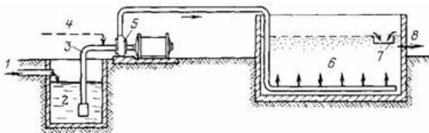
Сурет 4 - Ағынсыз флотацияға арналған құрылғының сызбасы 1-судың кіруі; 2-қабылдау резервуары; 3-соратын құбыр; 4-ауа құбыры; 5-су сорғыш; 6-флотациялық камера; 7-көбік жинағы; 8-тазаланған судың әкетілуі
